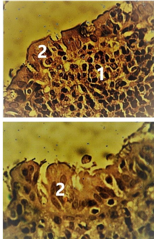
Рис. 2. Апікальні відділи лімфоїдних вузликів пейерових бляшок тонкої кишки. Парафінові зрізи; забарвлення за Ван-Гізоном; об'єктив 100: 1 – лімфоцитарні елементи; 2 – фолікул-асоційований епітелій
