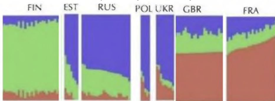
Мал. 2. Порівняння генетичної структури українців з іншими
