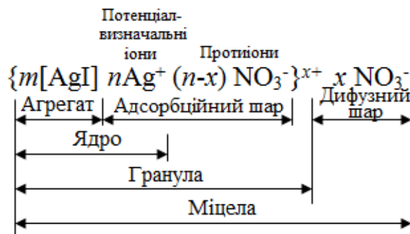
Формула міцели золю аргентум йодиду
